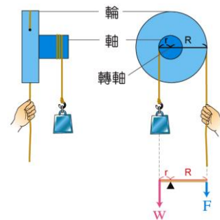
▲輪軸示意圖
